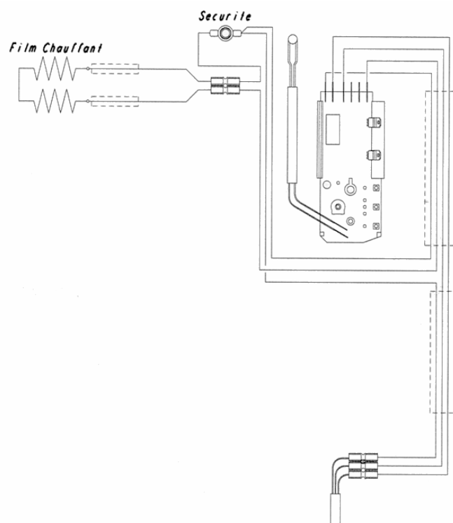
Version statique A68904.1/2
